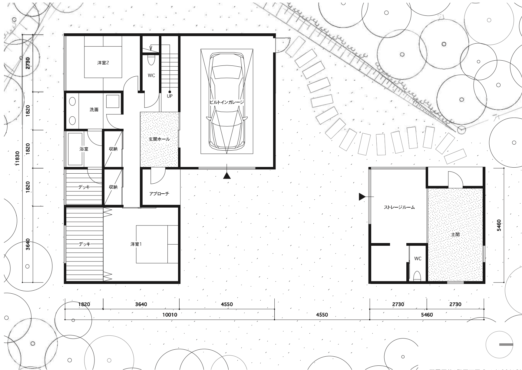
配置図兼1階平面図 S=1/100(A3)
