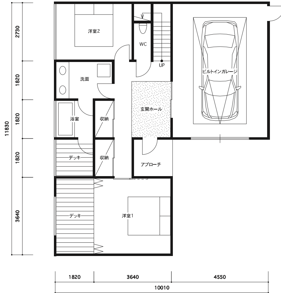
母屋1階平面図 S=1/100(A3)
