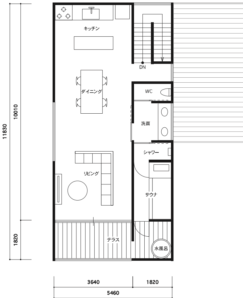
母屋2階平面図 S=1/100(A3)
