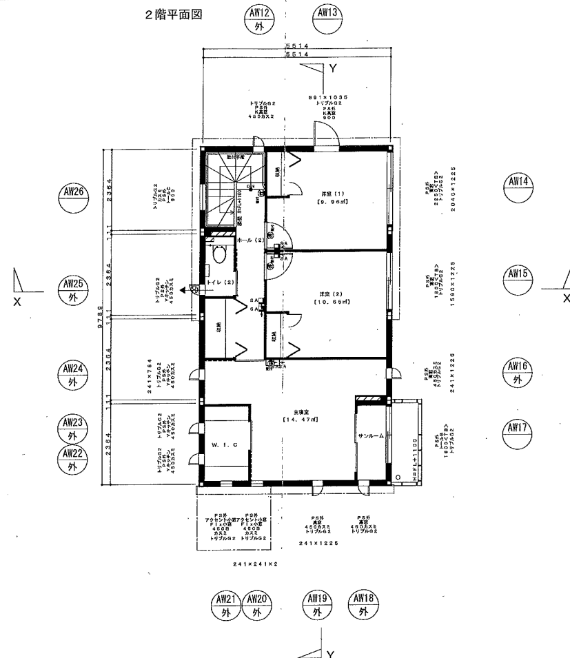
2階平面図
